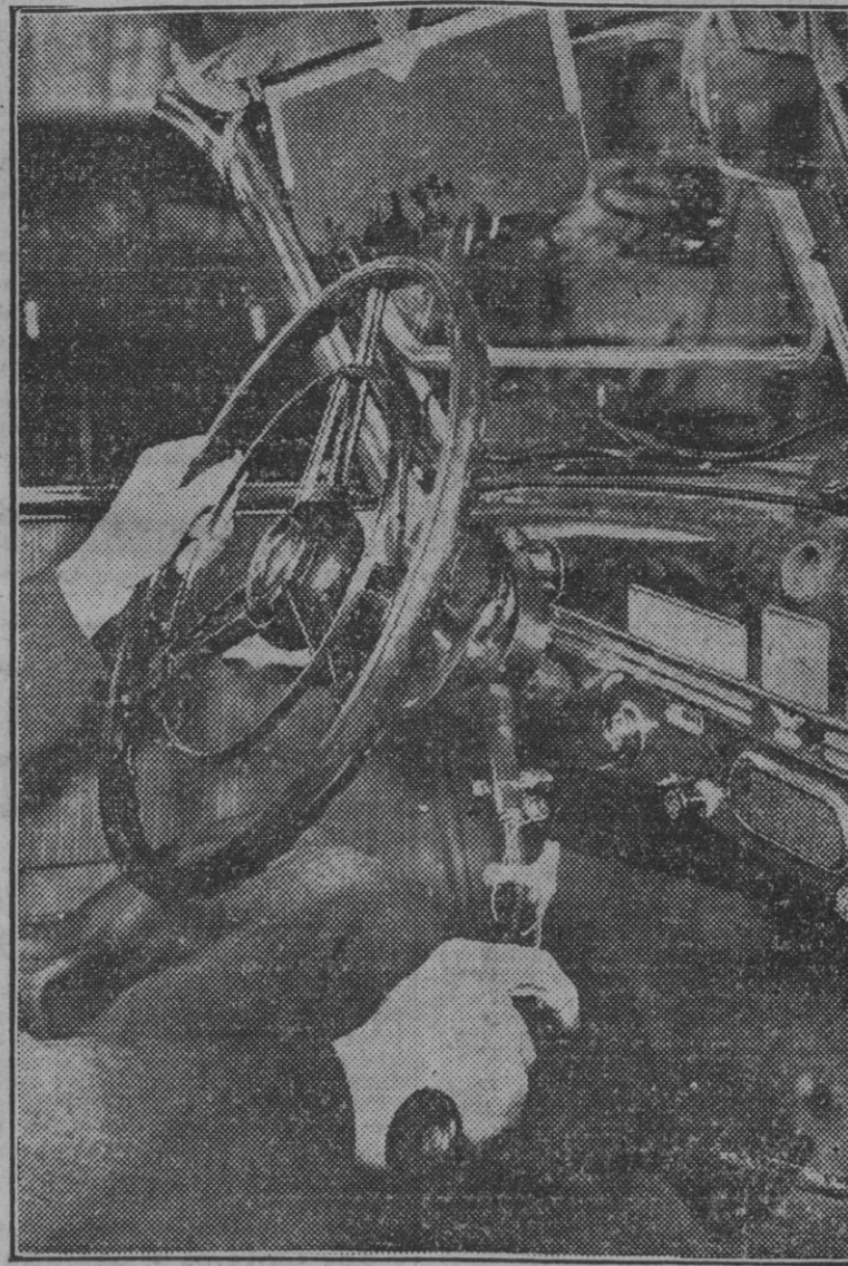
Por encargo de la Inspección de Sanidad del Ejército se ha creado un nuevo tipo de automóvil para los amputados o impedidos de las dos piernas. El freno y embrague se pueden manejar con las manos solamente. (Foto Hoffmann.)
