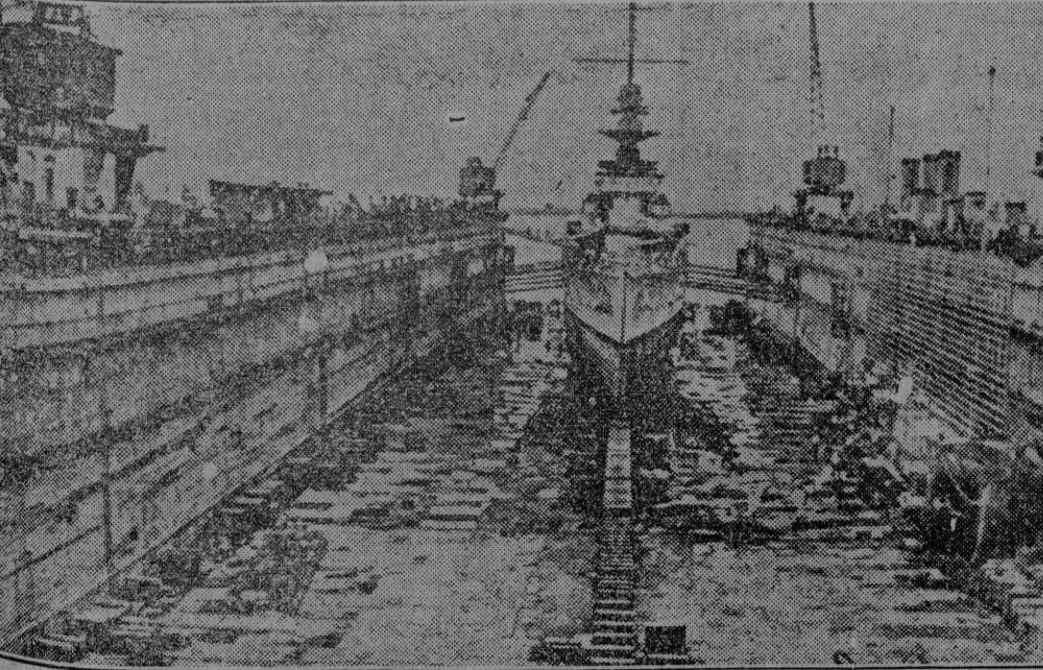
El dique flotante, de 50.000 toneladas, de Singapur, que, volado en parte por los ingleses, ha sido completamente destruido por los japoneses. (Foto Orbis.)
