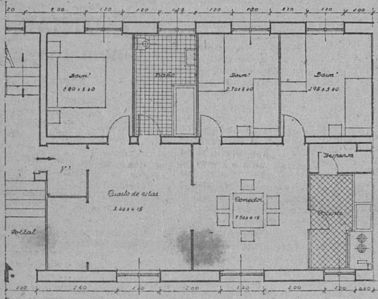
Plano de una de las viviendas
