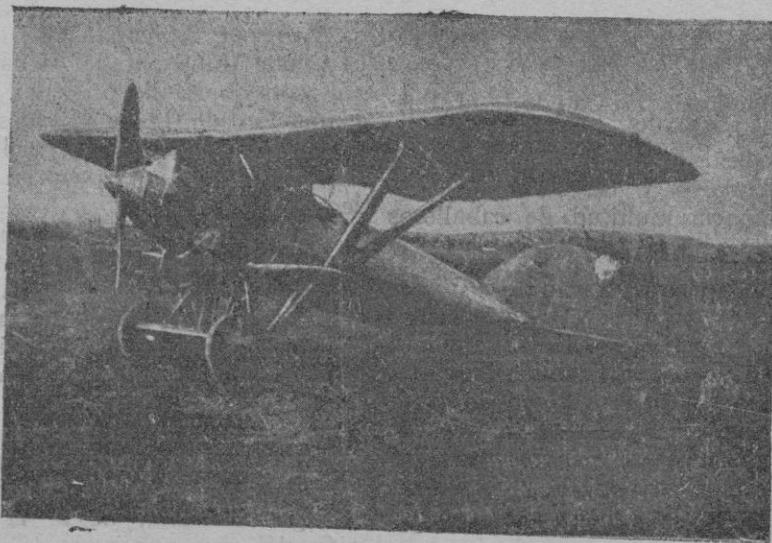
Guada'ajara.—Avión de caza, enteramente mecánico, primero de la serie que ha comenzado a entregarse a la aviación militar. Este aparato ha sido fabricado totalmente en España y alcanza una velocidad de 273 kilómetros por hora, pudiendo elevarse hasta una altura de 8,200 metros
