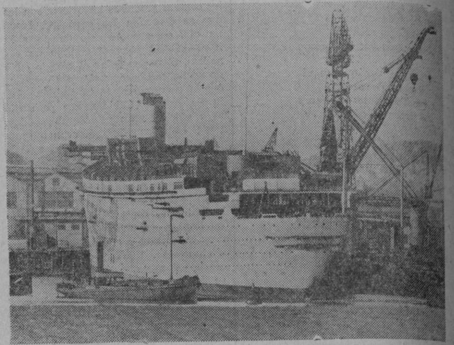
Los trabajos para la pronta terminación del gran paquebote de la «Cunard Line», «Queen Mary» se prosiguen activamente en Clydebank. La primera chimenea ha sido ya emplazada. Express-Foto.
