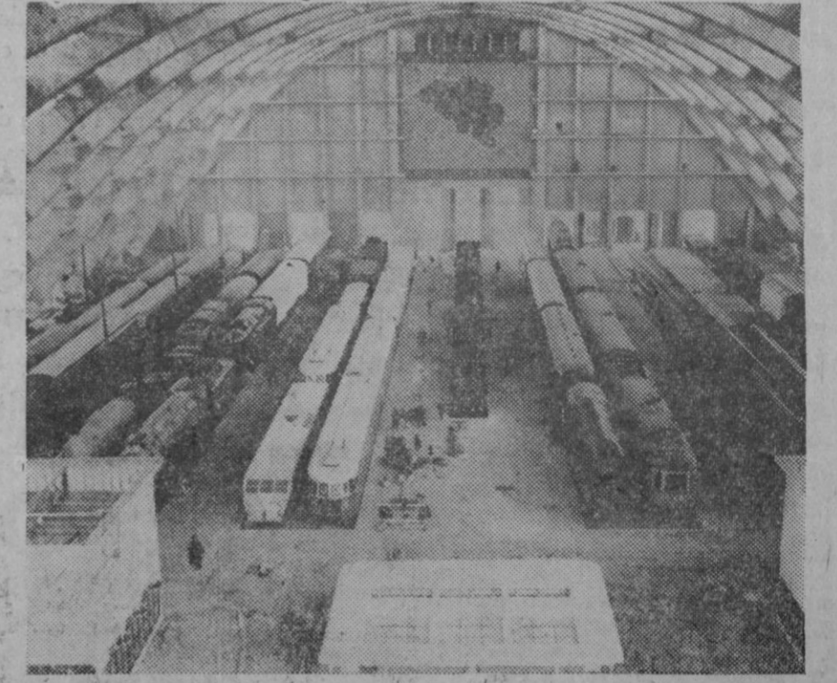
En la Exposición Internacional de Bruselas existe una estación en la cual se exhiben locomotoras, vagones y coches de la última construcción. (Express Foto).
