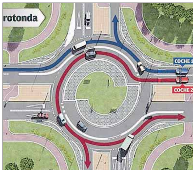
Infografía que muestra el funcionamiento de una turbo rotonda.
