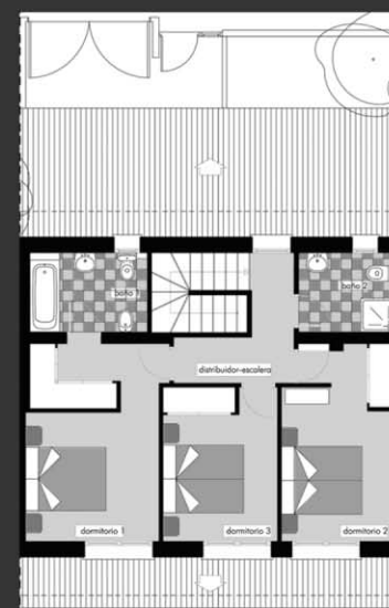
Planta primera
