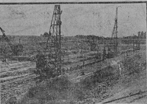
La machina con que se hace el hincado de las tablacas metálicas.
