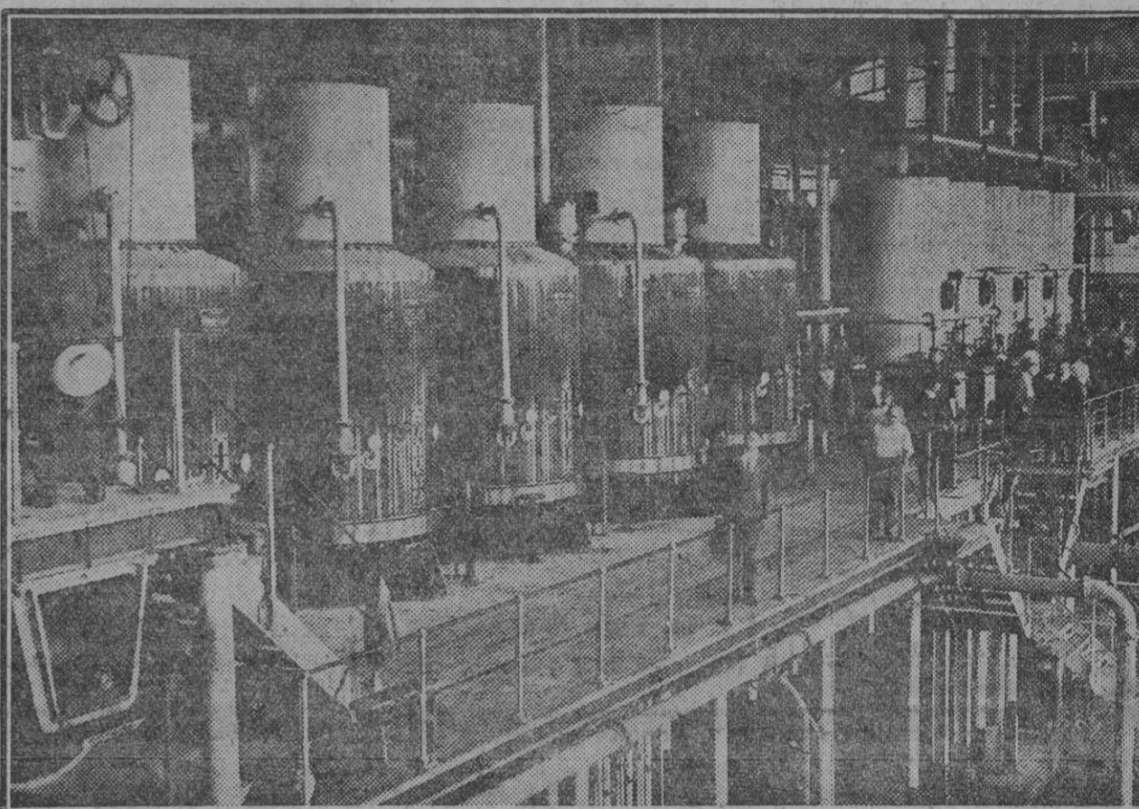
El quintuple y la carbonatación. Una de las naves de máquinas de la fábrica
