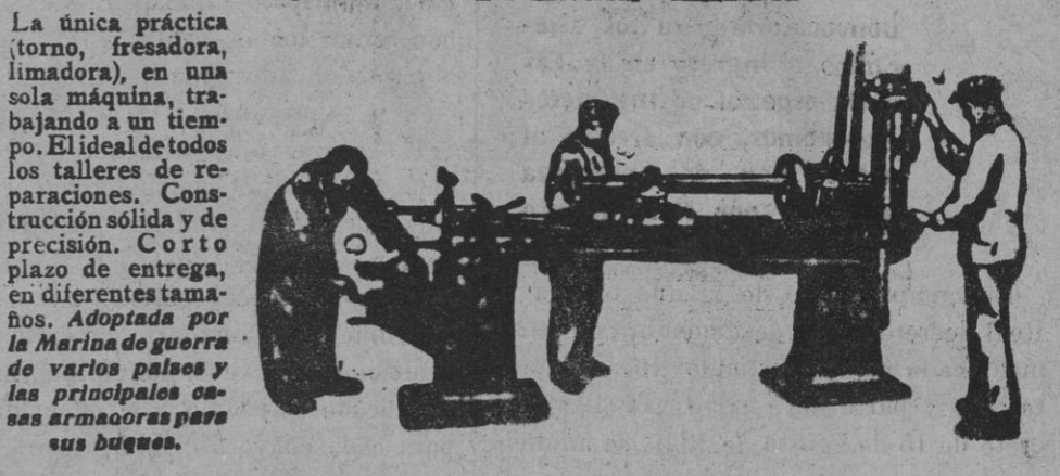
La única práctica (torno, fresadora, limadora, en una sola máquina, trabajando a un tiempo. El ideal de todos los talleres de reparaciones. Construcción sólida y de precisión. Corto plazo de entrega, en diferentes tamaños. Adoptada por la Marina de guerra de varios países y las principales casas armadoras para sus buques.
