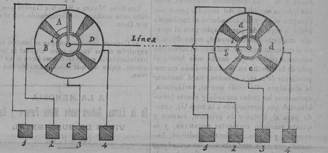
Fig. 1.—Esquema del montaje Baudot cuadruple.
