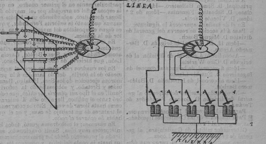
Fig. 2.—Transmisión y recepción.
