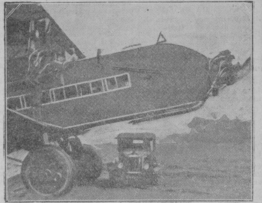
El nuevo aparato inglés de bombardeo que ha llamado la atención en toda Europa por las características de dicho aparato; como puede verse por debajo del tren de aterrizaje pasa sobradamente con holgura un auto de grandes dimensiones.
