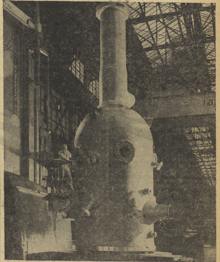
MOTOR LUNAR.— Los técnicos montan un motor F-1 en la fábrica que la North American tiene en Camoga, California. El motor está calculado para generar un empuje de 680.000 kilogramos. Un racimo de cinco motores F-1 integrará la primera fase del cohete Saturno V que se proyecta usar en el programa norteamericano Apolo de vuelo tripulado a la Luna. Esta fotografía ha sido tomada a través de una tobera de empuje del motor F-1
