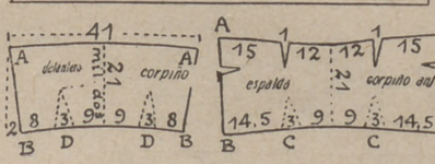
Croquis del patrón.
