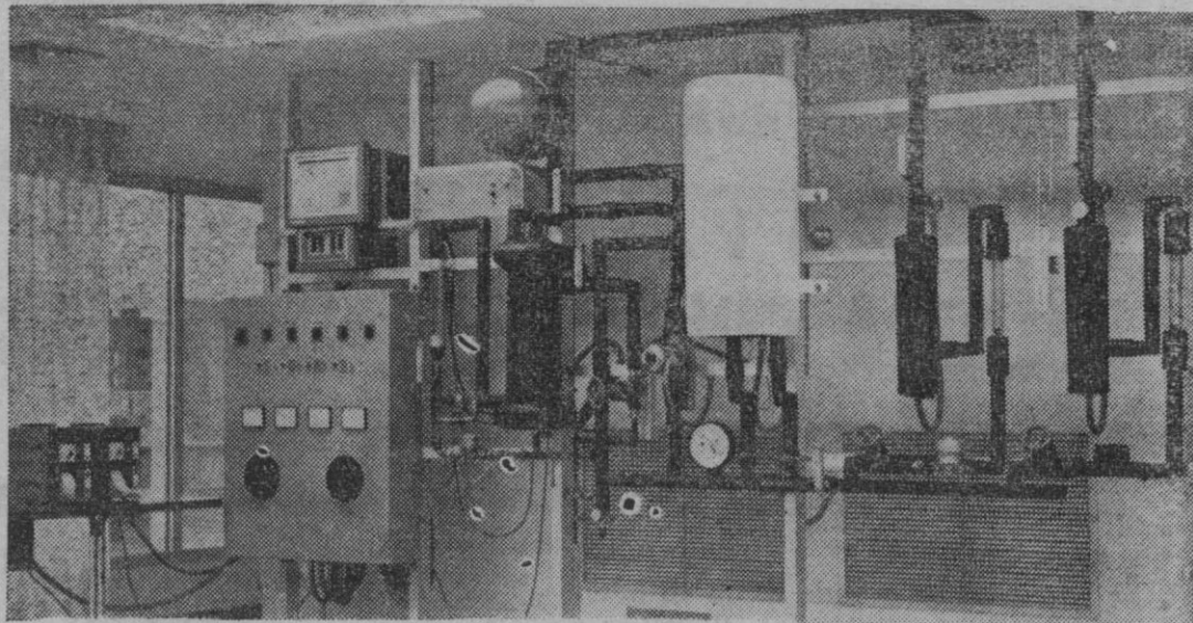
En el grabado, el laboratorio de ensayo de colectores, montado por GESA para la investigación y desarrollo de sistemas para la captación de energía solar.
