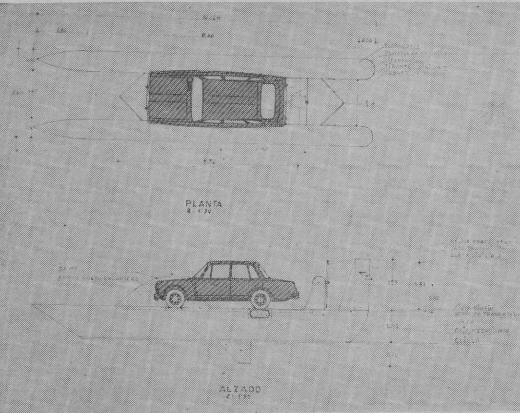
UNA PARTE DE LOS PLANOS DEL SR. FONT CATALA, INVENTOR DEL APARATO QUE CONVIERTE A LOS AUTOMOVILES NORMALES EN VEHICULOS APTOS PARA LA NAVEGACION, SIN NECESIDAD DE LA MAS MINIMA TRANSFORMACION.
