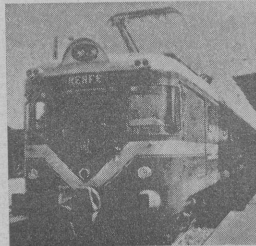
Los ha inaugurado el Ministro de Obras Públicas. Así son las unidades de los modernos electrotrenes que han entrado en servicio en la línea Caldas de Malavella-Sitges. Pueden alcanzar una velocidad de 140 kilómetros a la hora y reúnen adecuadas condiciones de comodidad.— (Cifra).
