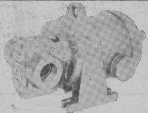
BOMBA DE ENGRANAJES SERIE EN Para trasiego de fuel, aceites, etc., Reversible
