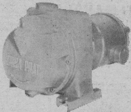
BOMBA CENTRIFUGA AUTOASPIRANTE SERIE CA Especial para elevar aguas sucias con cuerpos en suspensión
