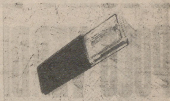
Proyector CIBIE halógeno H4 rectangular del modelo Seat Supermirafiori.
