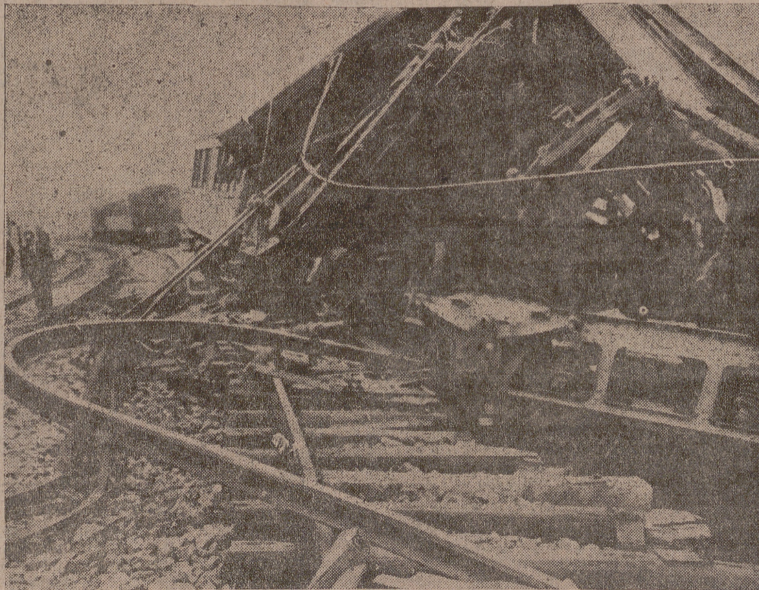
BARCELONA.—Estado en que quedó el tren eléctrico 1.204 de la línea Pobla de Segur a Barcelona, al descarrillar en una curva a la salida de la estación de Moncada. En el accidente se registraron tres muertos y sesenta y nueve heridos.—(Foto Cifra.)
