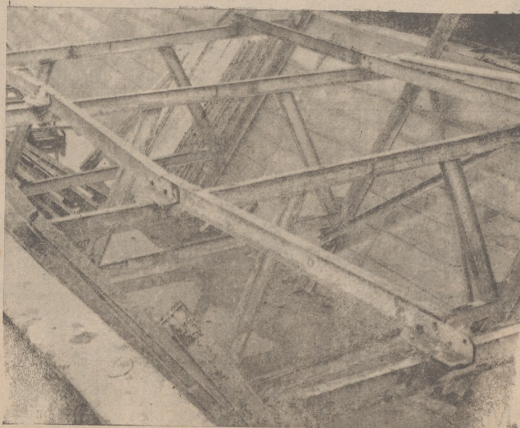
Uno de los aspectos del canal de la margen izquierda cuando esta en construcción
