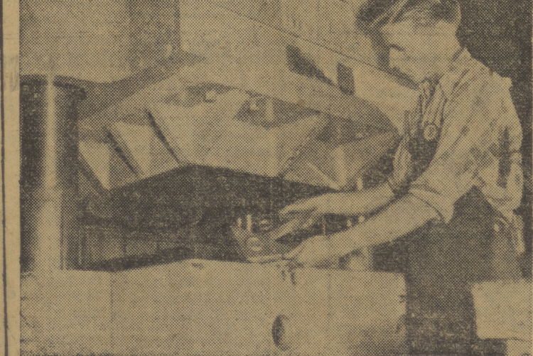
Un obrero muestra la pieza estampada y la matriz. Encima puede verse el bloque de caucho que hace la estampación.
