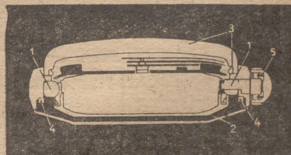
1 - JUNTA ELÁSTICA. 2 - FONDO DE ACERO ROSCADO. 3 - CRISTAL ARMADO. 4 y 5 - JUNTAS IMPERMEABLES.
