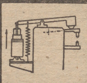
Máquinas de soldar por puntos.
