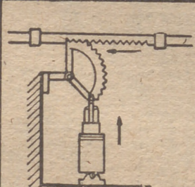
Accionamientos por cremallera.
