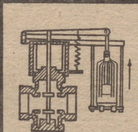
Válvulas para líquidos.
