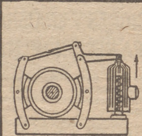
Freno y regulación.
