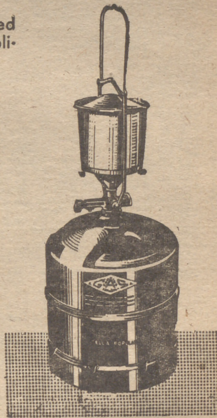
LUZ POTENTE CON BUTANO Para el campo y la ciudad Camping-Gas ha lanzado el LUMOGAS, aparato cómodo y manejable, que con una carga de butano de 26 pesetas de costo da luz potente (80 W) durante 75 horas y también garantizado el suministro de butano desde el momento de adquirir el LUMOGAS
