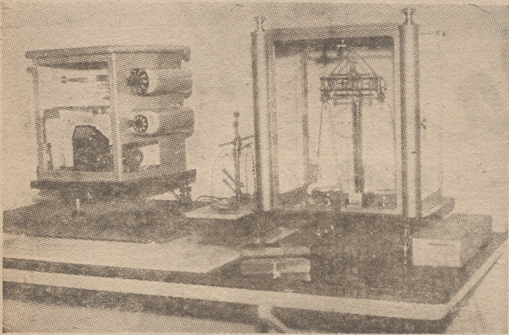
El peso electrónico, capaz de medir una millonésima de gramo. A su lado, la antigua balanza y un peso de milimetrada exactitud, tenido hasta ahora por el más moderno, hasta la llegada del electrónico. Tales son los nuevos elementos con los que el Laboratorio Municipal va contando para sus tareas analíticas.
