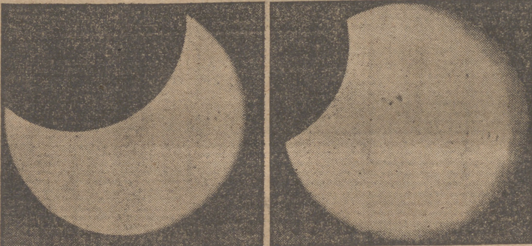
Estos dos gráficos muestran aspectos distintos del Sol durante dos fases del eclipse del astro rey el día 23 de noviembre. La foto de la izquierda fué tomada en el momento de máxima ocultación del Sol, a las doce horas y veintidós minutos. La segunda, a la una y treinta, cuando ya la sombra de la Luna es menor. En ambas se observan las manchas solares. Fueron obtenidas por el Servicio Naval Astronómico de Washington. (Fotos A. P.)
