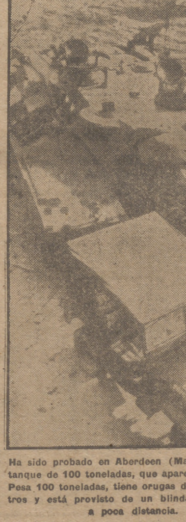
Ha sido probado en Aberdeen (Maryland) por primera vez este tanque de 100 toneladas, que aparece aquí al lado de un "jeep". Pesa 100 toneladas, tiene orugas dobles y cañón de 105 milímetros y está provisto de un blindaje especial para los asaltos a poca distancia. (Foto Citra.)
