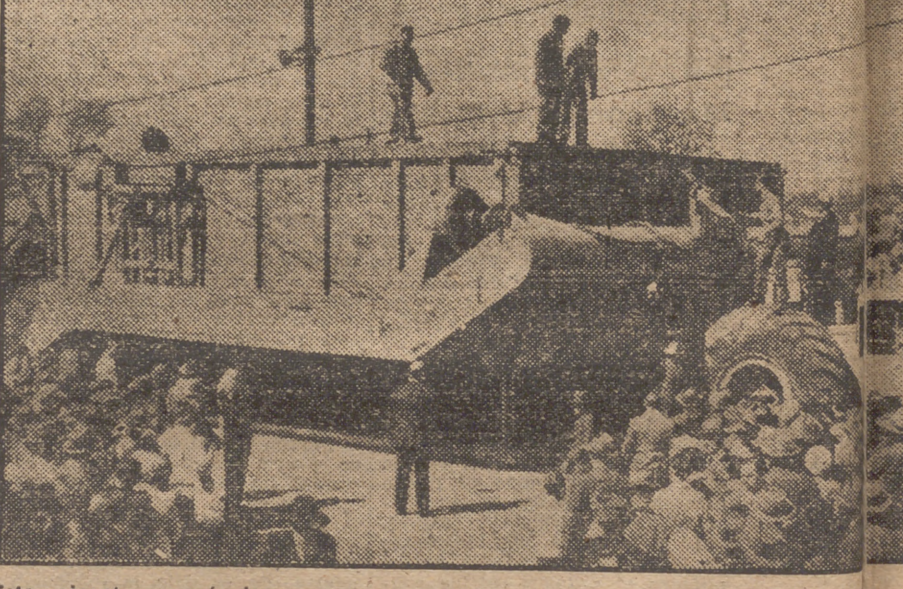
Esta gigantesca máquina, con sus enormes ruedas y con un peso de 165 toneladas, lleva dentro un modelo de casa de cuatro habitaciones. Es llenada de cemento y a las veinticuatro horas, seco el cemento, la casa, de una pieza, está hecha, y la misma máquina, llamada "Biddy", la transporta y va a colocarla en el terreno preparado al efecto. Arriba: la máquina en plena acción; abajo: la casa que ha salido de sus entrañas. Puede fabricar también casas de dos pisos, y hasta con sótano. El precio de la que aquí se ve, incluidas instalaciones eléctricas, agua, pintura, etc., es de 2.600 dólares. El inventor de las "Biddy" las alquila a los contratistas de construcción por la bonita renta mensual de 11.000 dólares.
