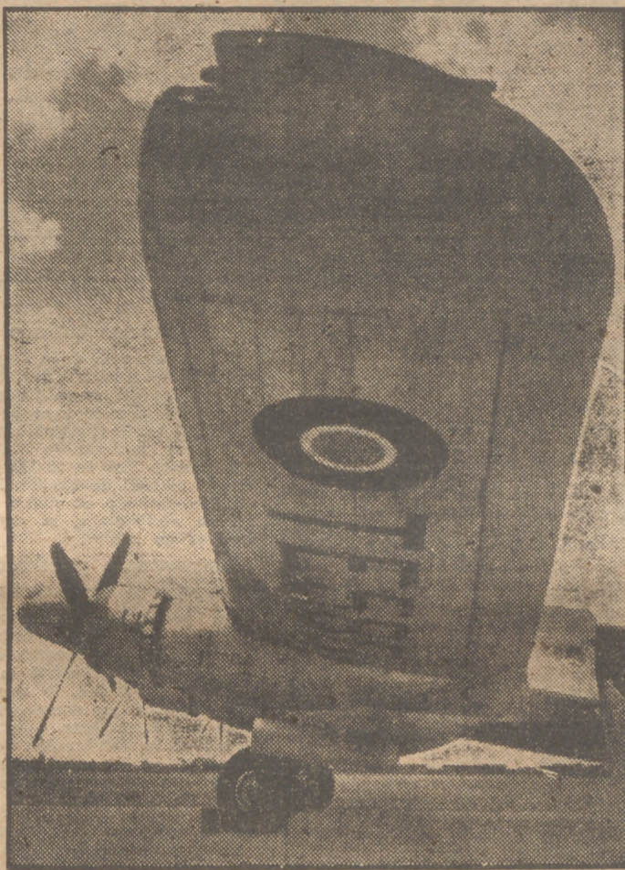
Handley Page es un nombre de abolengo en la historia de la aviación mundial. Ahora la gran marca inglesa ha lanzado este nuevo avión de transporte destinado a las líneas que unirán la metrópoli con los Dominios. Sus características son: Velocidad de crucero, 300 millas por hora; techo, a esa velocidad y con 75.000 libras de carga, 22.700 pies; cuatro motores de 1.675 HP. Bristol Hércules; refrigeración por aire; motores radiales; capacidad, de 34 a 50 pasajeros; el largo de las alas es de 113 pies.
