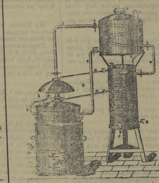
Nuevo alambique destilador.
