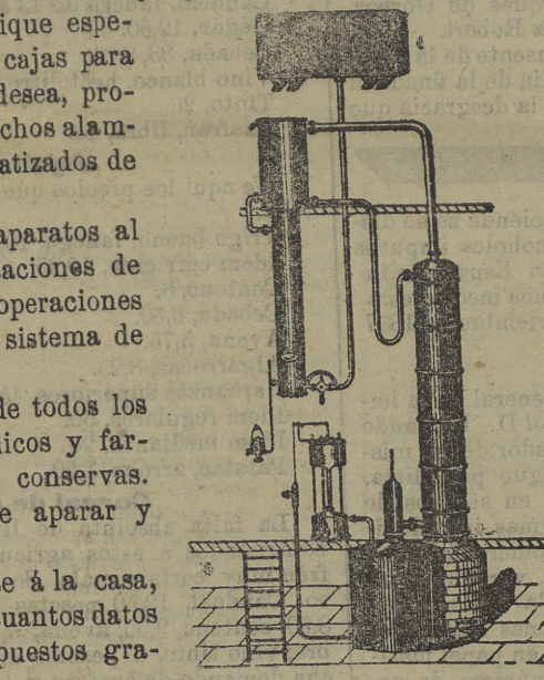
Aparato de rectificación.
