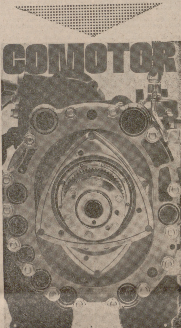
Investigaciones tratan de resolver los problemas de estanqueidad de estos sistemas, cuestión decisiva en la realización del actual motor rotativo.
