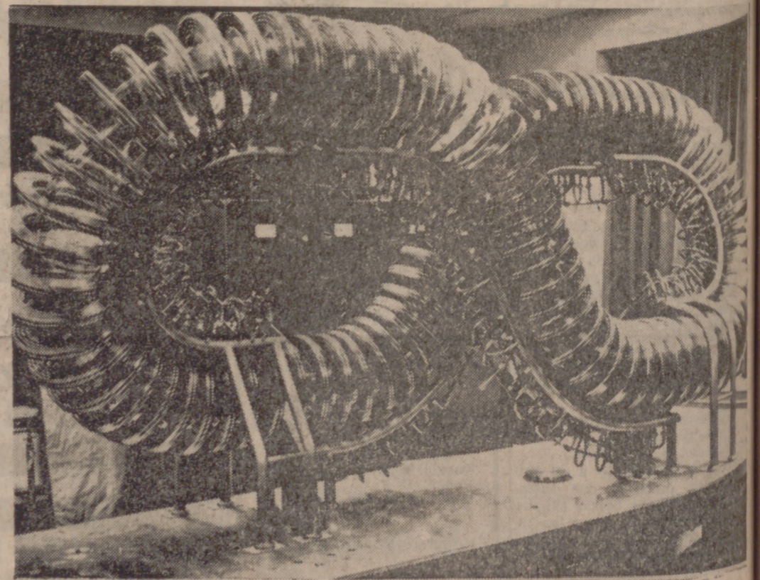
Un ingenioso dispositivo en forma de ocho que sirve para almacenar hidrógeno a temperaturas elevadísimas y estudiar las posibilidades de utilizar comercialmente el fenómeno de fusión nuclear.
