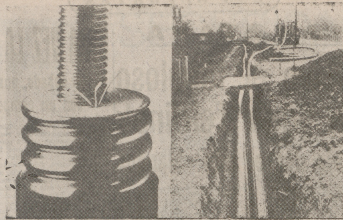
HANNOVER.—El cable para calefacción a distancia es de cobre en el interior y de acero en el exterior, y se enrolla flexiblemente. Se puede tender en el fondo del mar. La construcción permite el transporte de gases.
