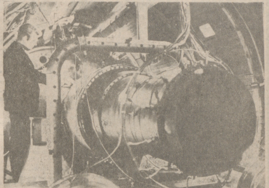
STUTTGART.—(Dad).—El que en el terreno universitario del Pfaffenwald, de Stuttgart, se encuentra el único banco de pruebas de altura del mundo para turbopropulsores, lo saben sólo los iniciados. Está a la disposición, tanto de la investigación internacional como de la industria y sirve para el estudio del comportamiento de funcionamiento de turbopropulsores y de turbohélices, así como de sus elementos de construcción bajo condiciones diferentes. En la celda de ensayo, de diez metros de largo y tres metros de diámetro, se pueden simular velocidades de vuelo de hasta el 1,1 de la velocidad del sonido (número Mach 1,1) en el suelo y hasta el número Mach 2,4 a 20 kilómetros de altura de vuelo. La temperatura de aspiración del grupo motopropulsor se puede variar por medio de refrigeradores previos, turbinas de refrigeración y calentadores de aire, entre 70° negativos y 200°C positivos. Para la aspiración de los gases de escape se dispone de tres compresores de un total máximo de 10.000 kilovatios de potencia de accionamiento. Nuestra foto muestra un grupo motopropulsor "Orfeo" en la celda de ensayo.
