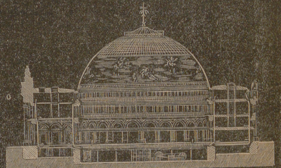
Chauffage par aero calorifère.
