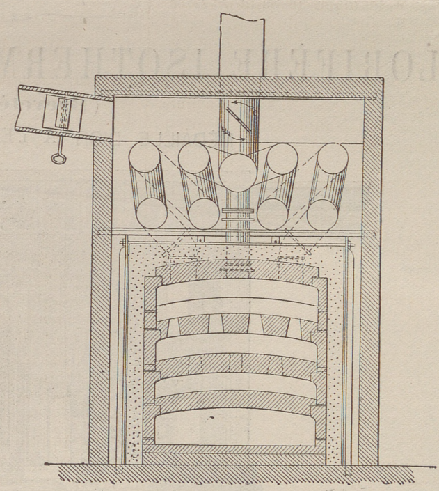
Fig. 2 - Coupe transversale
