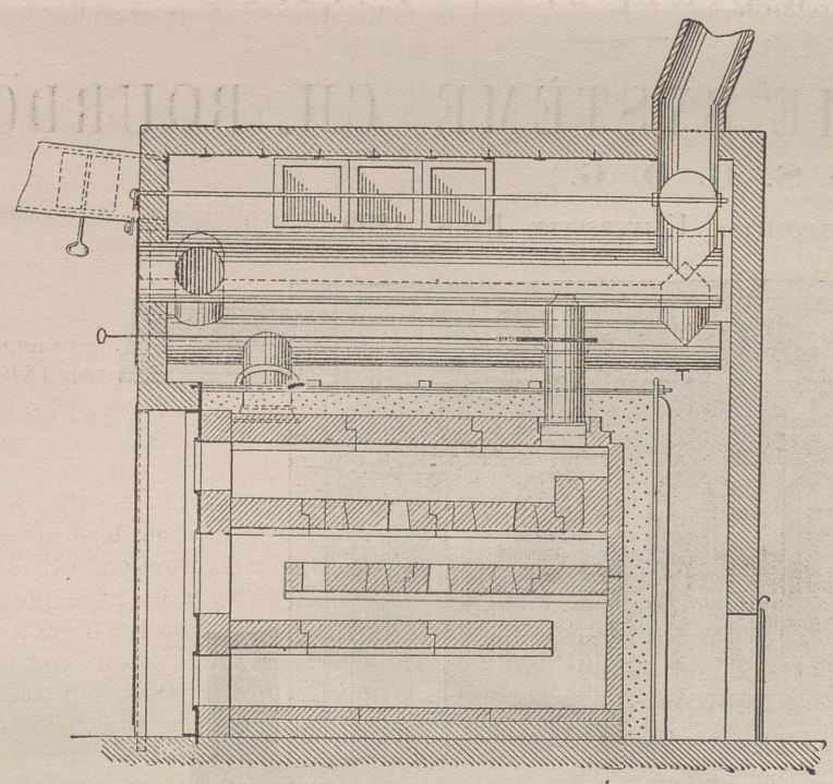
Fig. 1 - Coupe longitudinale
