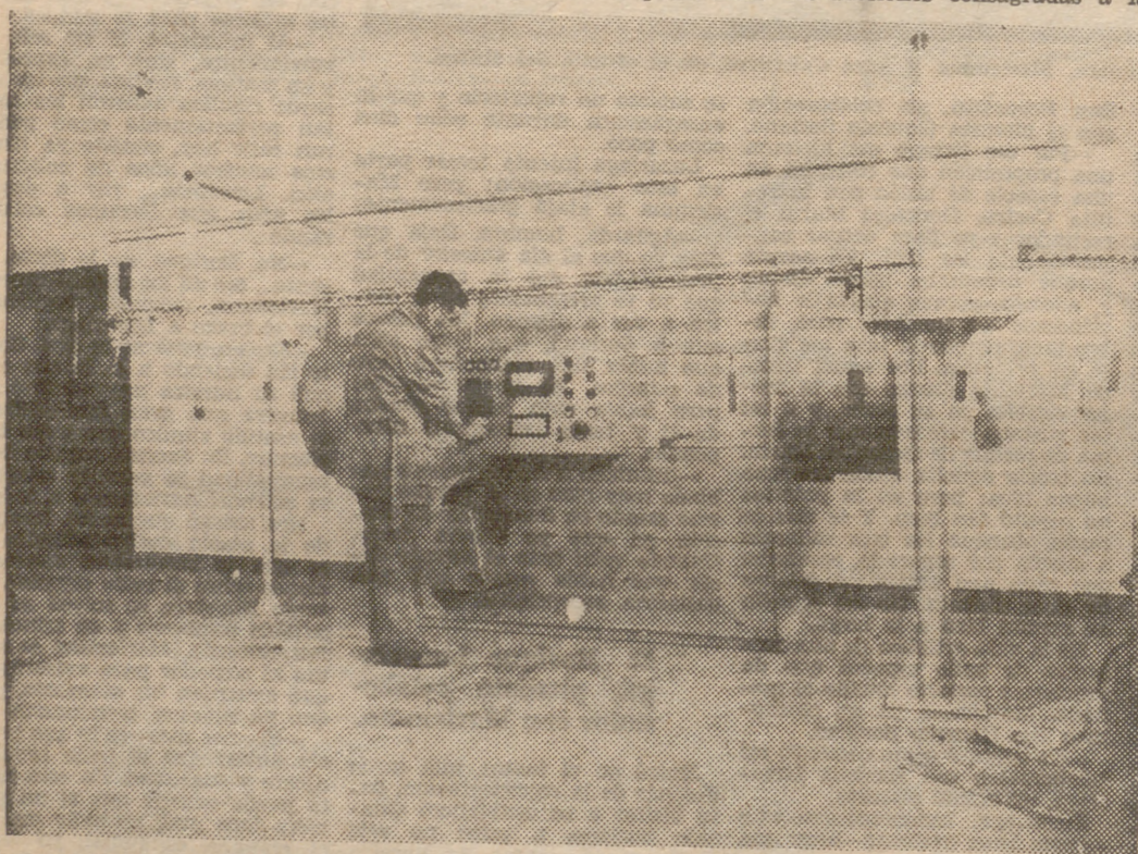
Sección de Aplicación. Túnel de secado automático, en cadena, por rayos infrarrojos
