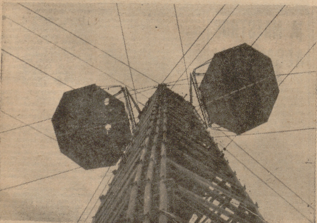
REFLECTORES PASIVOS
