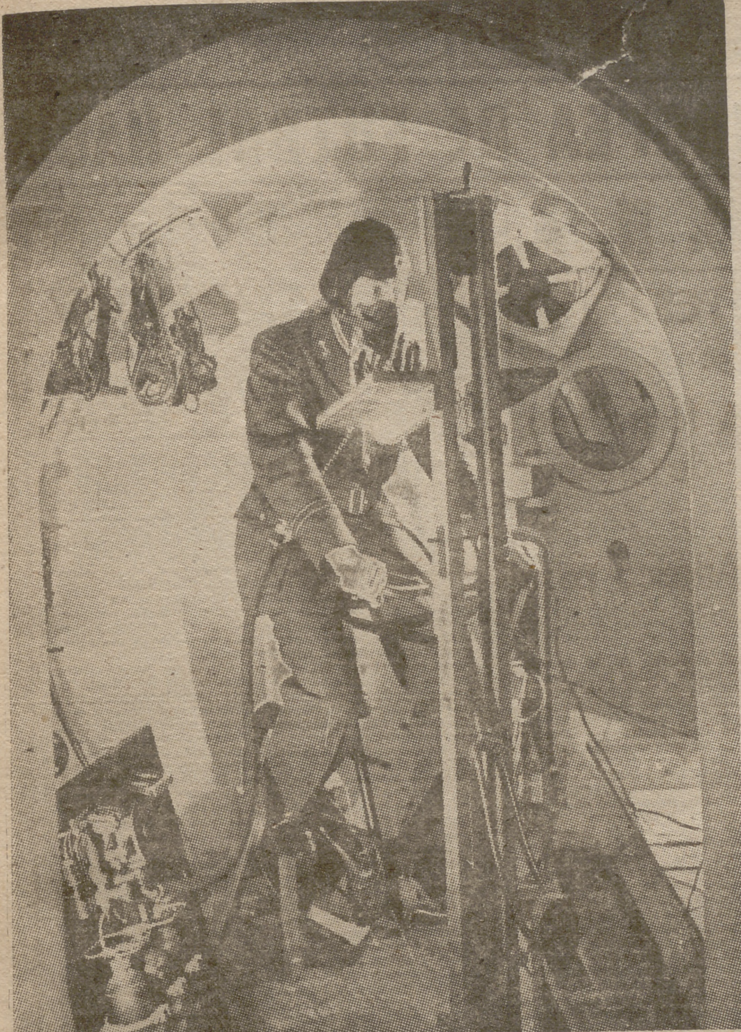
Una serie de aparatos registran las reacciones de los pilotos mientras éstos están sometidos a esfuerzos físicos violentos. Este chasis de bicicleta dispone de un sistema de fricción regulable, a fin de que el piloto tenga que realizar mayores o menores esfuerzos. (Foto Europa.)
