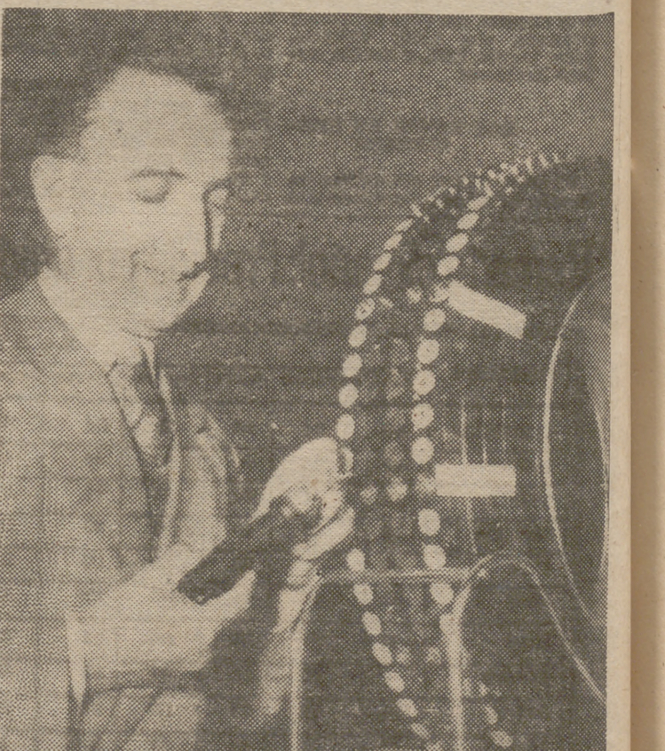
Un ingeniero belga ha ideado este tipo de neumático con «teclas» metálicas intercambiables que, al mismo tiempo que evita los patinazos, prolonga su duración, economizando materia prima y divisas
