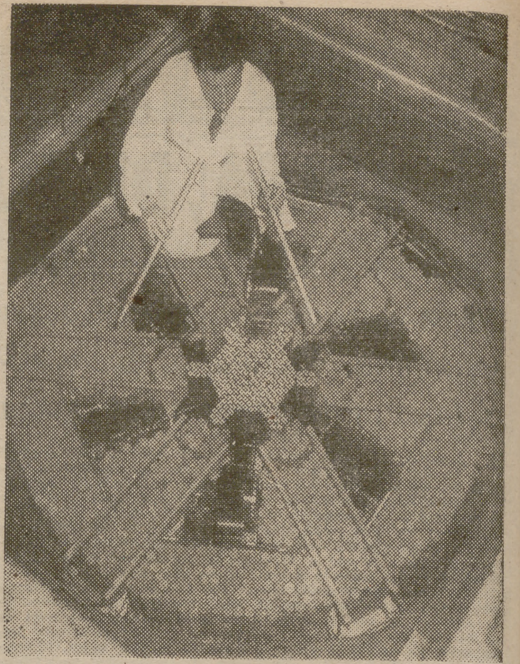
Colmena atómica de un reactor, vista desde arriba.
