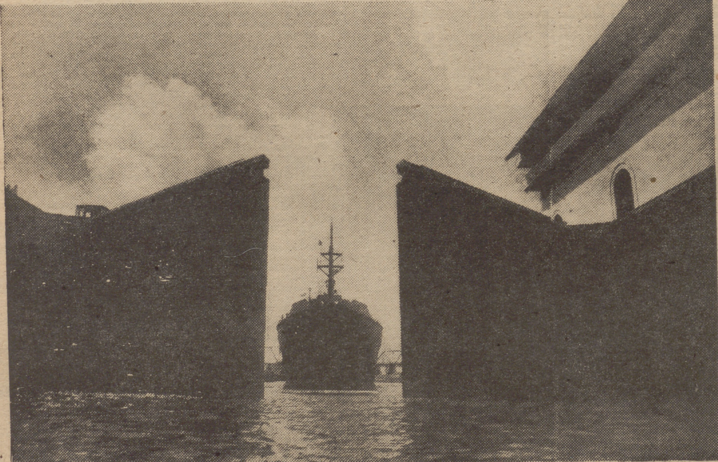
Momento de abrirse las esclusas de Miraflores para el paso de un buque hacia el Atlántico
