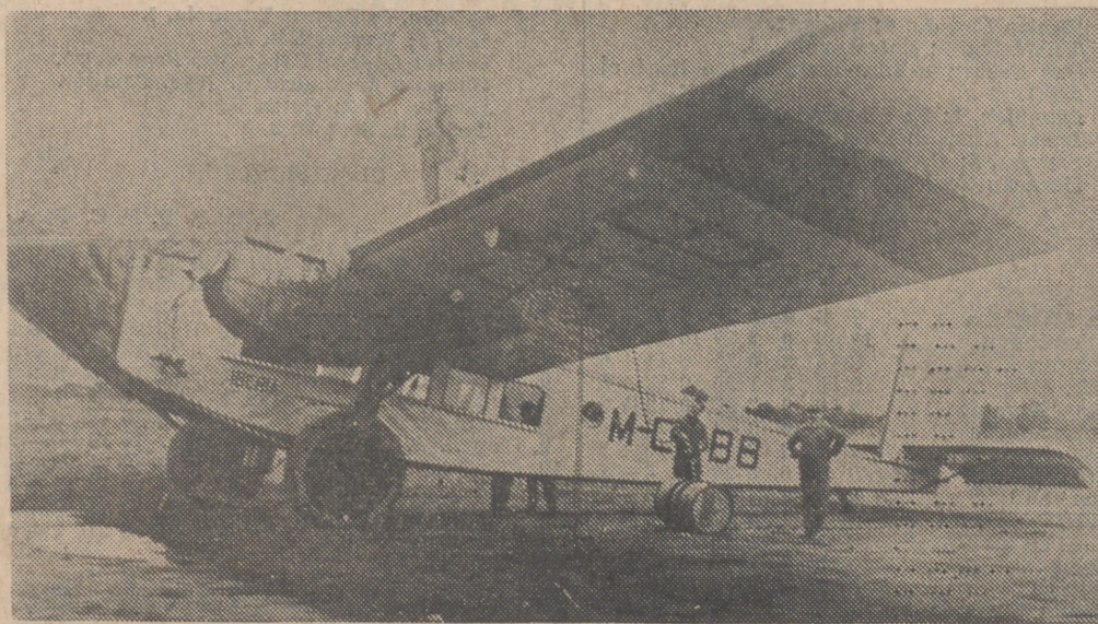
Trimotor "Rohrbach VIII-Roland", que volaba en 1927. Su velocidad era de 170 kilómetros por hora, con tres motores "3 BMW-IV" de 260 HP, peso de 7.250 kilos y envergadura de 26 metros. Era capaz para diez pasajeros
