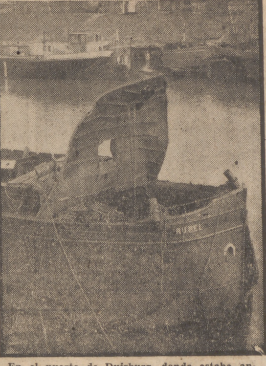
En el puerto de Duisburg, donde estaba anclado este barco holandés — el «Rupel» —, se produjo un trágico accidente que costó la vida al hijo del patrón del buque. Una botella de gas metano hizo explosión, y aparte de la desgracia personal ya señalada, dejó al barco en el estado que recoge la foto
