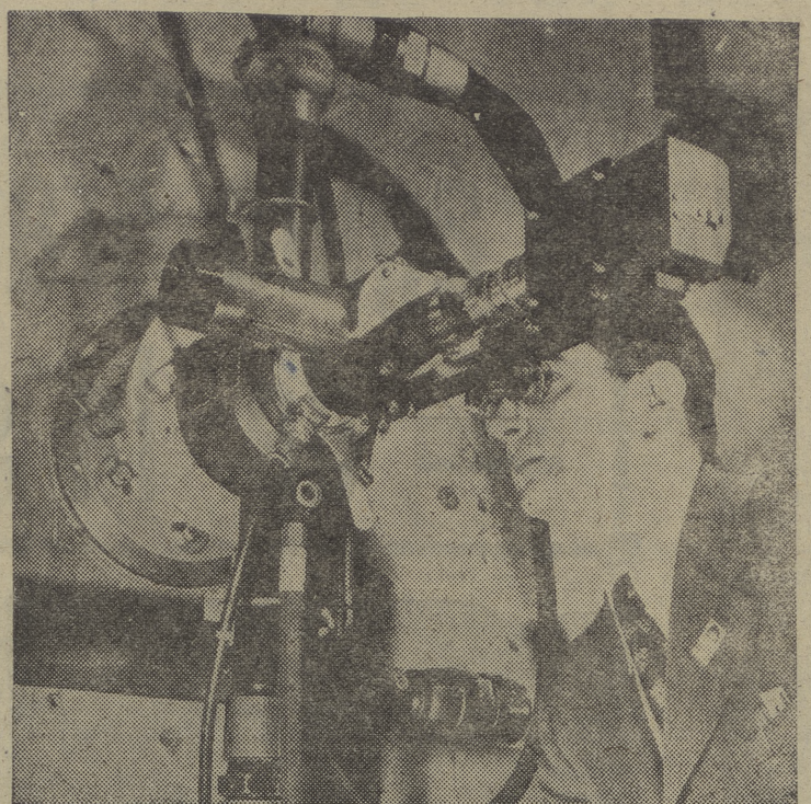
Una cámara cinematográfica (a la derecha del observador), va tomando fotografías en color sobre el desarrollo de una turbina de gas en Nueva York. El ingeniero de la General Electric sigue las incidencias a través de un periscopio especial que se va enfriando por medio de agua.
