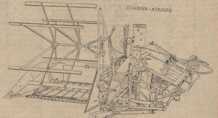
Cada faena agrícola cuenta ya con la maquinaria propia para ayudar y hacer más llevadera la tarea del hombre. Los dibujos pormenorizan el complicado mecanismo de una segadora-atadora y una agavilladora
