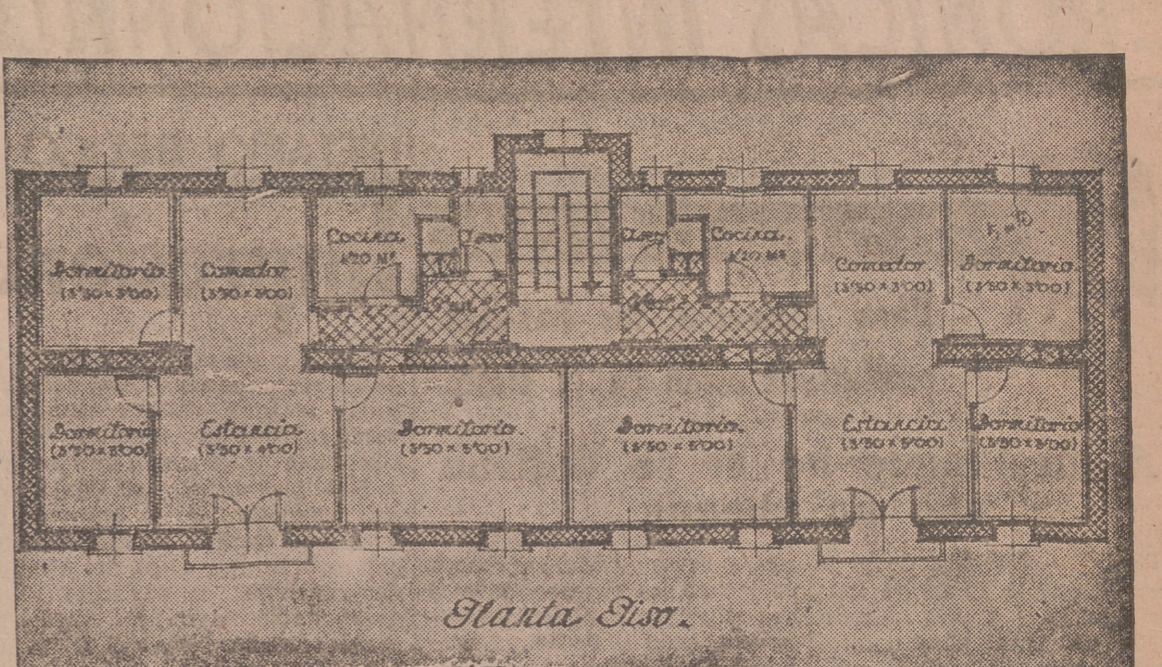
Planta del grupo de viviendas cuya construcción comenzó ayer
