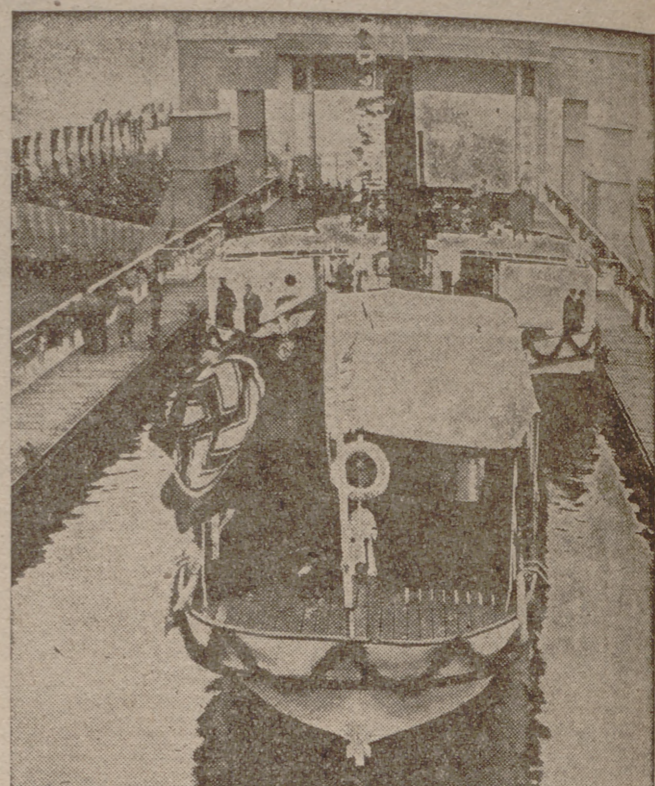
UN NUEVO CANAL DE NAVEGACION A TRAVES DE ALEMANIA.—El elevador de buques "Magdeburg-Rothensee" ha sido inaugurado por el ministro del Reich, Hess. Así se ha abierto a la explotación la gran vía navegable Rhein-Oder, a través del Reich.
