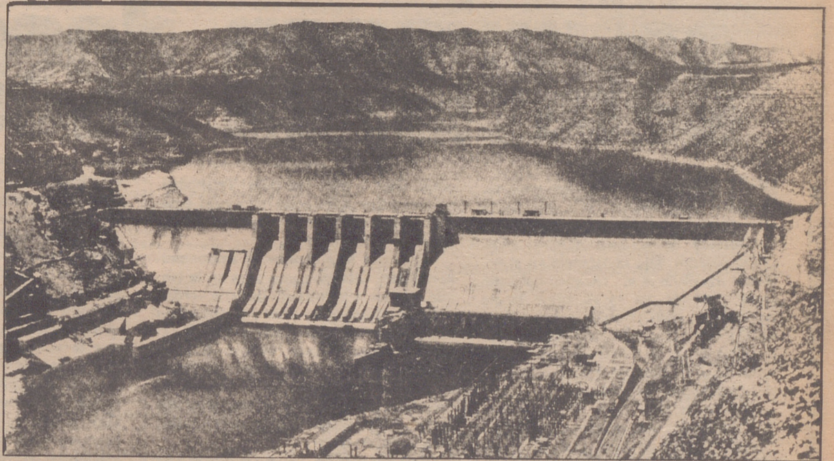
Impresionante perspectiva de la presa de Mequinenza levantada 2 kilómetros aguas arriba del encuentro del Ebro con el Segre, en el límite de Catalunya con Aragón. Construida entre 1958 y 1964, con una altura de muro de 80 metros, da origen a un lago artificial de cerca de 100 kilómetros de longitud capaz de almacenar 1.530 millones de metros cúbicos de agua y regular el caudal en el curso inferior.
