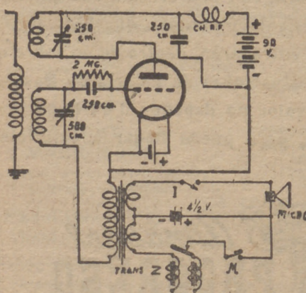
Figura 185.—Emisor radiotelefónico radiotelegráfico
